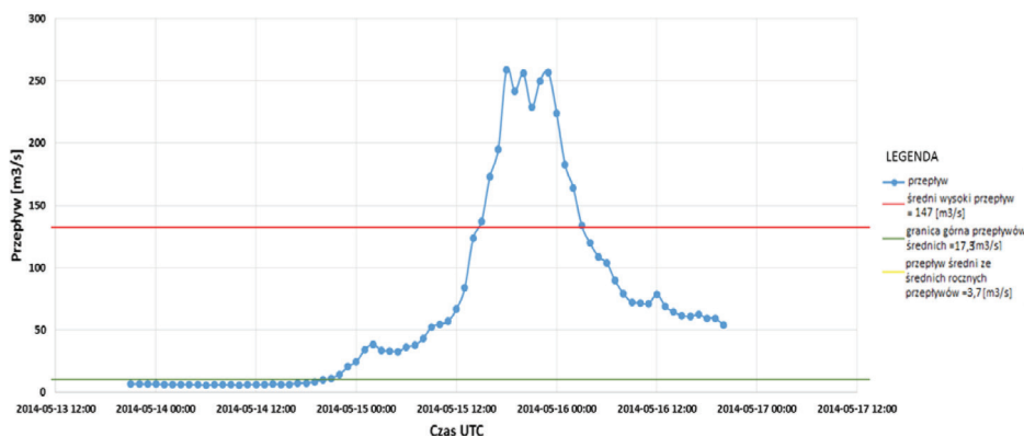
Rysunek 2. Hydrogram przepływu rzeki Kamienica Nawojowska ( www.pogodynka.pl )
