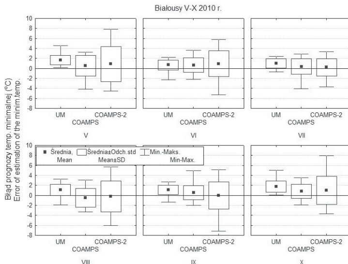
Rysunek 2. Średni dla poszczególnych miesięcy bezwzględny błąd prognozowania minimalnej temperatury dnia. Białousy V–X 2010 r. Figure 2. Mean absolute error of forecasting of minimal day temperature for consecutive months. Białousy V–X 2010
