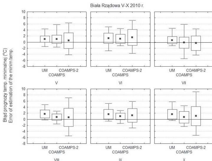
Rysunek 3. Średni dla poszczególnych miesięcy bezwzględny błąd prognozowania minimalnej temperatury dnia. Biała Rządowa V–X 2010 r. Figure 3. Mean absolute error of forecasting of minimal day temperature for consecutive months. Biała Rządowa V–X 2010
