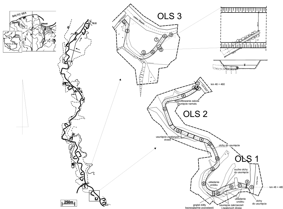
Rysunek 1. Lokalizacja starorzeczy objętych projektem renaturyzacji oraz zakres zaplanowanych prac hydrotechnicznych Figure 1. Localisation of oxbow-lakes to be restored and the scope of hydrotechnical treatments
