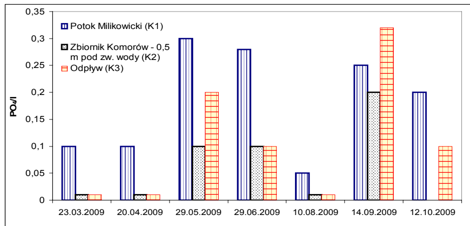
Rysunek 4. Stężenie PO 4 -3 w wodzie z terenu zbiornika Komorów w 2009 r. Figure 4. Phosphates concentration in water from Komorów reservoir in 2009
