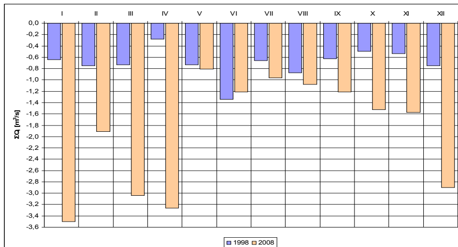
Rysunek 3. Suma użytkowania zasobów wodnych na wodowskazie Zgorzelec w 1998 r. i 2008 r.
