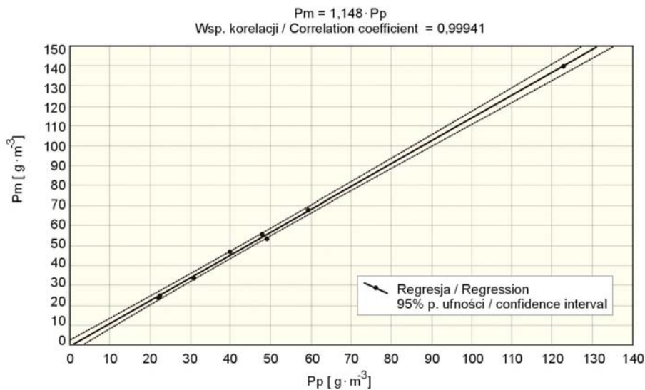
Rysunek 5. Zależność regresyjna pomiędzy koncentracją zmaczenia w przekroju ( P_m ) a koncentracją zmaczenia w punkcie ( P_p ) ustalona dla rzeki Łęg Figure 5. Regression relation between concentration of suspended sediment in section ( P_m ), and concentration of suspended sediment in point ( P_p ), established for the River Łęg
