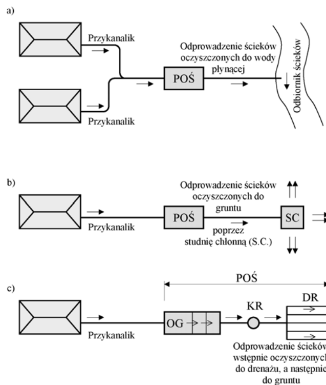
Rysunek 1. Unieszkodliwianie ścieków z zastosowaniem przydomowych oczyszczalni ścieków (POŚ): a) z odprowadzeniem ścieków oczyszczanych do wody płynącej, b) i c) z odprowadzeniem ścieków oczyszczonych do gruntu [Heidrich i in. 2008] POŚ – przydomowa oczyszczalnia ścieków, SC – studnia chłonna, OG – osadnik gnilny, KR – komora rozdziału, DR – drenaż rozsączający
