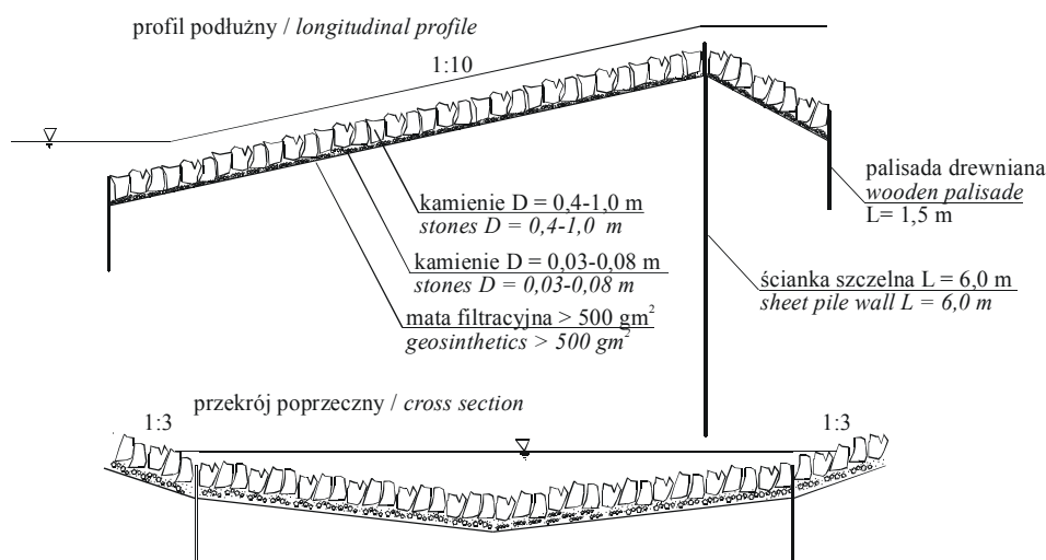
Rysunek 19. Schemat modelu bystrza na rzece Böhme w Fallingbostel, zabezpieczonego przed rozmyciem ściankami szczelnymi z palisad i stalową ścianką na progu Figure 19. Model draft of the rapid hydraulic structure constructed in the Böhme River in Fallingbostel; palisades and steel sheet pile walls prevent scour of the structure
