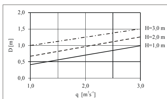
Rysunek 18. Wykres doboru wielkości kamieni na płycie bystrza, oznaczenia: D – wielkość kamieni naturalnych [m], q – przepływ jednostkowy [ \text{m}^2\text{s}^{-1} ], H – wysokość bystrza [m]
