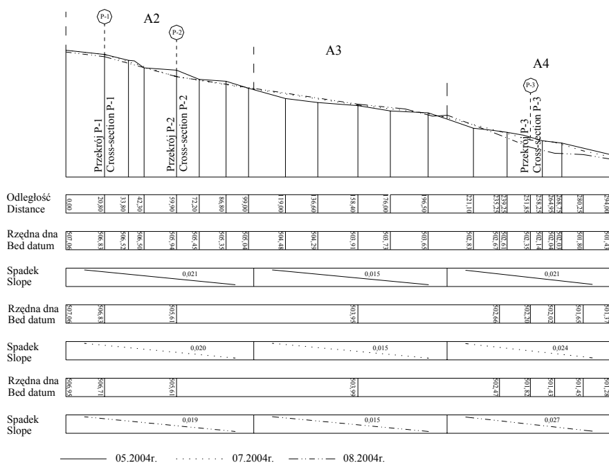
Rysunek 2. Profil podłużny potoku Słomka Figure 2. Longitudinal profile of the Słomka stream
