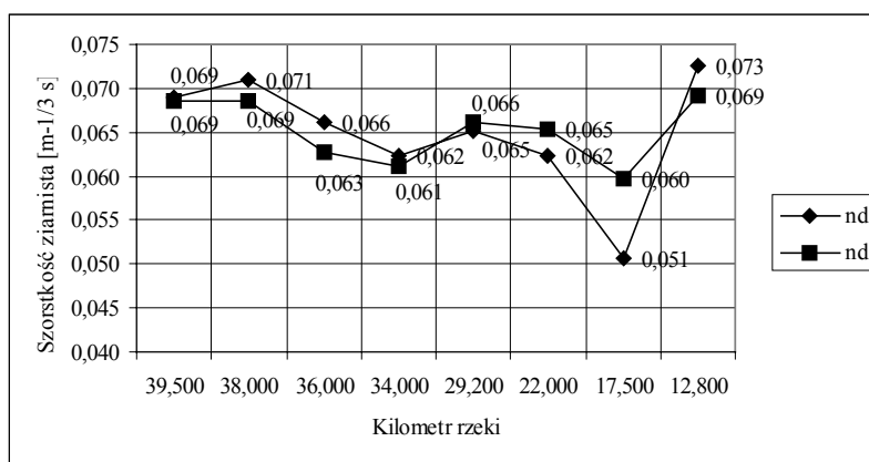
Rysunek 4. Przebieg zmienności współczynnika szorstkości ziarnistej
