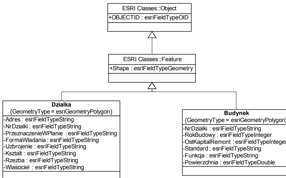
Rysunek 1. Diagram struktury statycznej UML – klasy obiektów i ich atrybuty Figure 1. UML static structure diagram – object classes and their attributes
