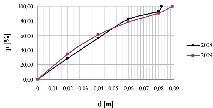
Rysunek 5. Krzywe uziarnienia – próby z bystrza
