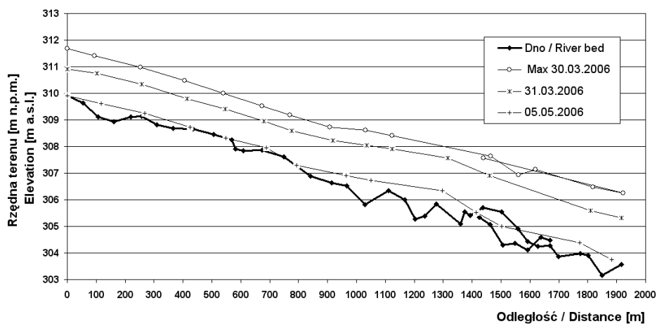
Rysunek 4. Poziom zwierciadła wody na badanym odcinku rzeki Skawy Figure 4. Measured water surface level on a section of the Skawa River
