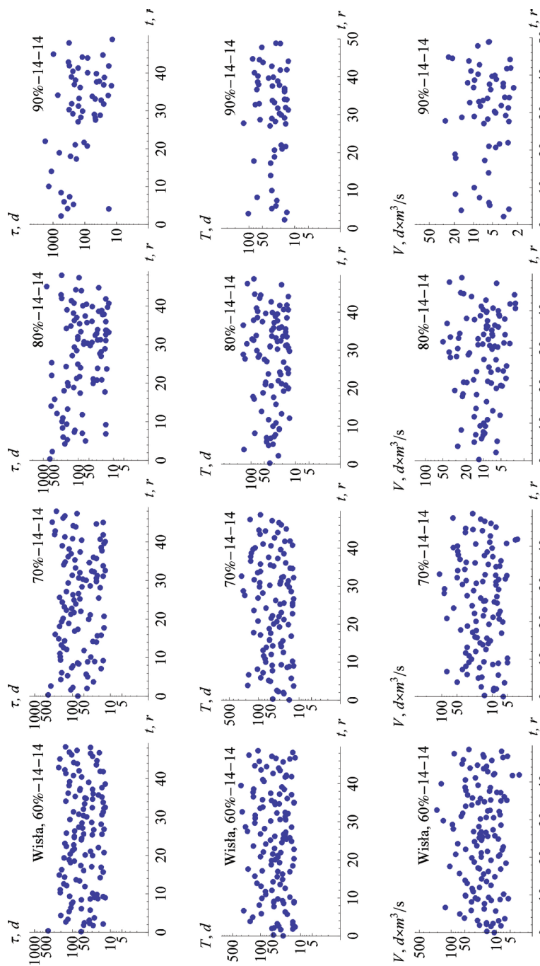
Rysunek 4. Szeregi czasowe czasów \tau pomiędzy kolejnymi niżówkami, czasów trwania niżówki T oraz deficytów niżówki V w zależności od początku t niżówki ( r oznacza rok) dla zadanych wartości względnego średniego w roku czasu p przekroczenia przepływu progowego Q_p i przyjętych wartości (T_{min}, \tau_{min}) .
