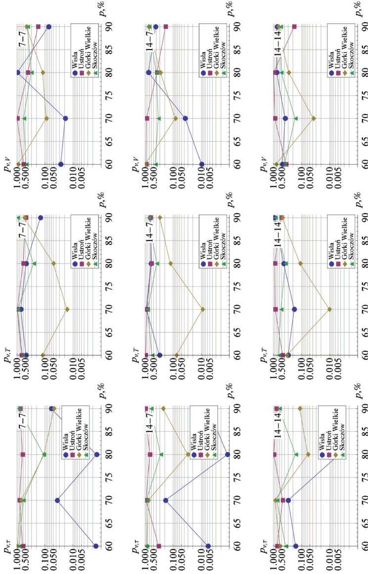
Rysunek 5. Wartości p_v testu hipotezy H_0(a=0) o stacjonarności szeregu czasowego czasów \tau pomiędzy kolejnymi niżówkami, czasów T trwania niżówki oraz deficytów V niżówki w zależności od względnego średniego w roku czasu p przekroczenia
