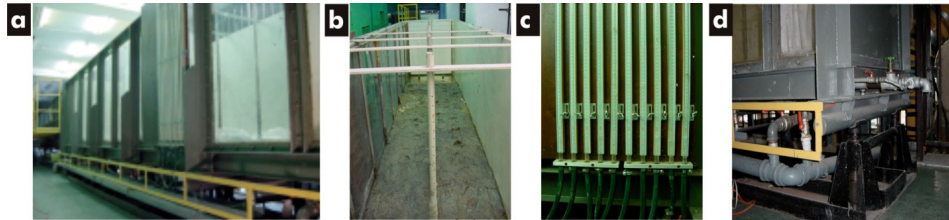
Rysunek 1. Średniowymiarowy aparat do badania filtracji przez modele nasypów: a) widok ściany czołowej, b) wnętrze aparatu z ilowym uszczelnieniem przydennym, c) tablica pomiarowa do odczytu poziomu wody w piezometrach, d) zawory pomiarowo-upustowe
