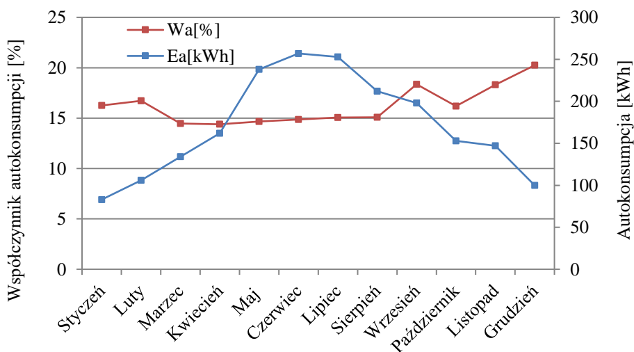
Rysunek 1. Przebieg zmian współczynnika autokonsumpcji oraz ilości energii zużytej w procesie autokonsumpcji w układzie miesięcznym w roku 2022 Figure 1. The course of changes in the self-consumption coefficient and the amount of energy used in the self-consumption process on a monthly basis in 2022
