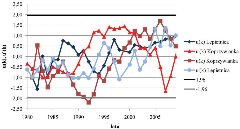
Rysunek 1. Wyniki testu MKS z 95% przedziałem akceptacji dla przepływów maksymalnych w zlewniach Lepietnica i Koprzywianka [źródło: opracowanie własne]
