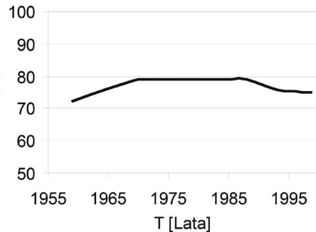
Rysunek 3. Zmienność szerokości koryta Soły w przekroju Żywiec w latach 1959-1999.
