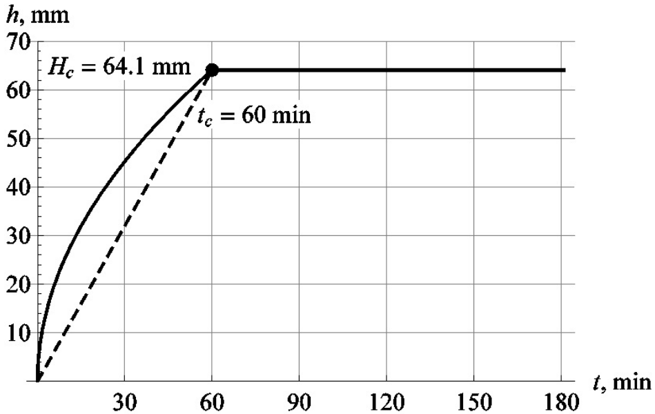
Rysunek 3. Model Chomicza (linia ciągła) przebiegu czasowego wysokości opadu h(t) (pokazany dla opadu nr 3 z 7 lipca 1861 r., tabela 1) od początku opadu do zmierzonego czasu trwania t = t_c (punkt) i przedłużonego do chwili t_{max} = 180 minut, gdyż jego wysokość h = H_c przekracza wszystkie wysokości H_{c,min} opadu z tabeli 2. Linia przerywana oznacza linię średniego natężenia opadu.
