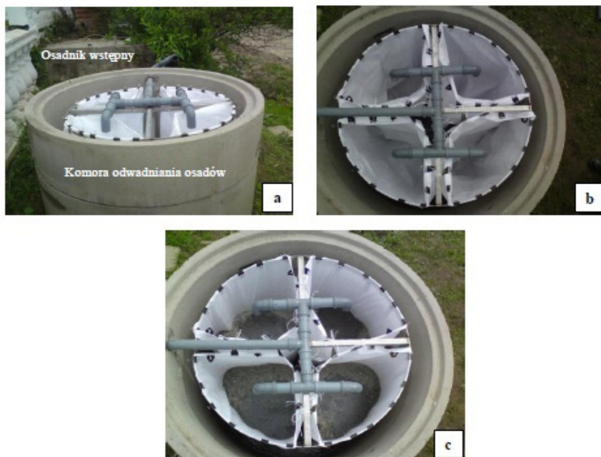
a – widok z boku, b – widok z góry (przed napełnieniem worków osadem), c – widok z góry (po napełnieniu worków osadem) a – side view, b – view from the top (before filling the bags of sediment) c – view from the top (after filling the bags of sediment)
