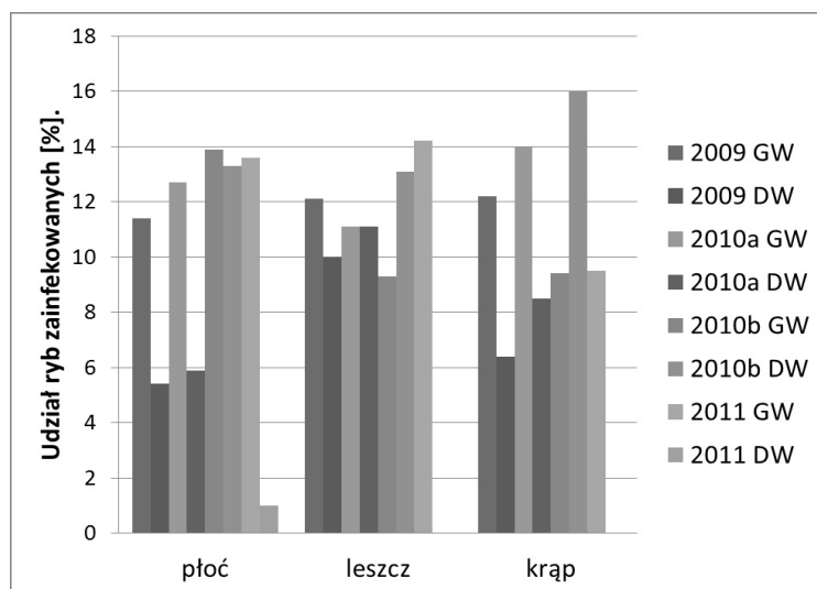
Rysunek 1. Procentowy udział ryb chorych w poszczególnych populacjach [%] Figure. 1. Percentage of infected fish in the various populations [%]
