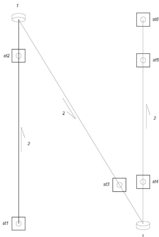
Rysunek 6. Baza łamana do wyznaczenia stałej dodawania w GLM Figure 7. Polyline calibration base to determine prism constant at GLM
