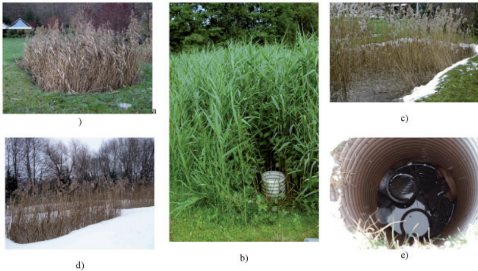
Fotografia 1. Złóża gruntowo-roślinne w Paszkowie, widok oraz elementy konstrukcji, a-złóże 2, b- wylot z osadnika na złożo 1, c- złożo 4 widok w zimie, d – eksploatacja w zimie, e – studzienka rozdzielcza [fot. Katarzyna Paweńska]
