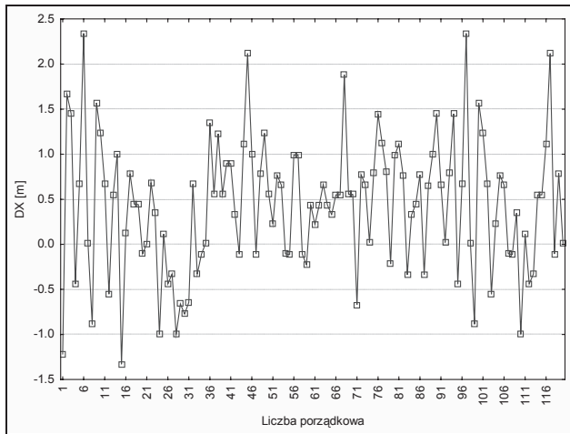
Rysunek 3. Wyniki błędów pomiarów stacjonarnych rzędnej [H] na punkcie 2041 Figure 3. The results of measurement errors fixed for ordinate [H] at the point of 2041
