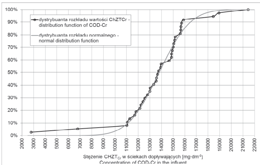
Rysunek 6. Dystrybuanta rozkładu wartości \text{ChZTCr} na dopływie oczyszczalni oraz rozkładu normalnego o najmniejszym błędzie średniokwadratowym aproksymacji wartości \text{ChZTCr}
