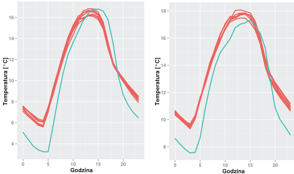
Rysunek 4. Temperatury przewidywane przez model UM (krzywe czerwone) i temperatury zmierzone (krzywa niebieska) w kwietniu (panel lewy) i maju (panel prawy) 2009 roku, Dąbrowice
