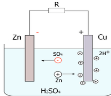
Rysunek 1. Ogniwo Volty – jedno z najprostszych ogniw galwanicznych skonstruowane i opisane w 1790
