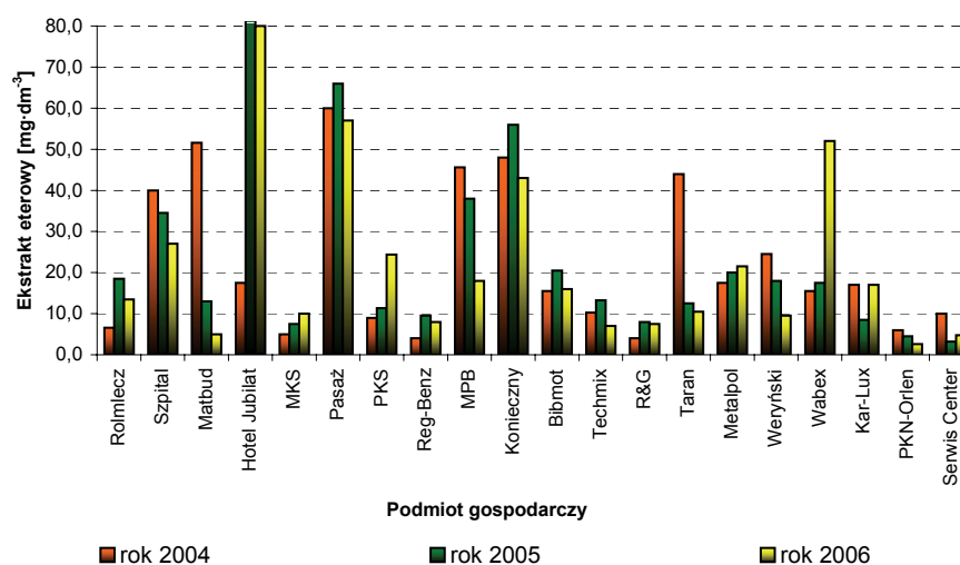
Rysunek 6. Wielkość ekstraktu eterowego w ściekach odpływających z poszczególnych podmiotów gospodarczych w latach 2004–2006
