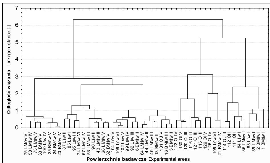
Rysunek 6. Aglomeracja metodą Warda (oznaczenia jak na rys. 1) Figure 6. Agglomeration using the Ward method (denotations as in fig. 1)
